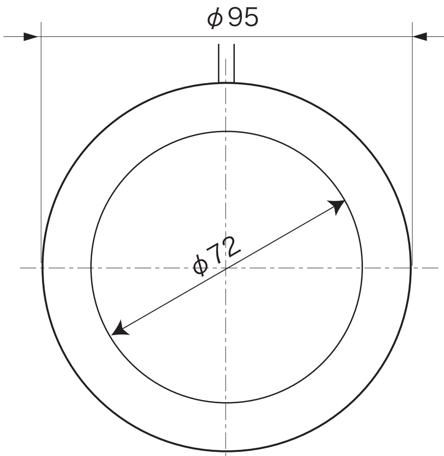
円形ステージ型 LED 透過照明 RL95 寸法図
